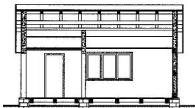
Фиг. 6. Надлъжен разрез на къщичката на Стоянка Илиева.
