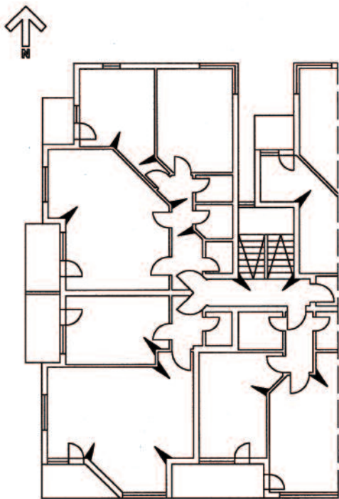
Фиг. 5. Съвременно архитектурно решение. Изобилие от вътрешни ръбове.
