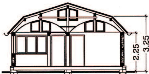
Фиг. 4. Къщичка на Стоянка Илиева. Вертикален разрез.
