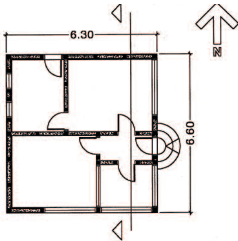
Фиг. 3. Къщичка на Стоянка Илиева. Разпределение.
