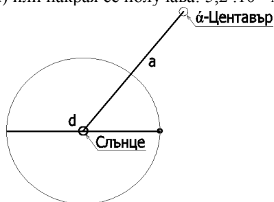
фиг.1 Строеж на Слънчевата система
