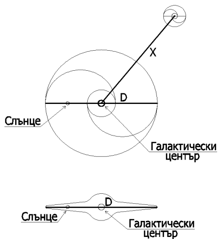
фиг.2 Строеж и напречен разрез на Галактиката
